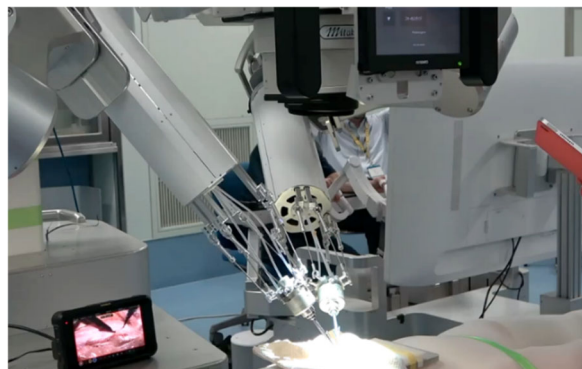
参考図 2 九州大学で開発中のマイクロサージェリーロボット
